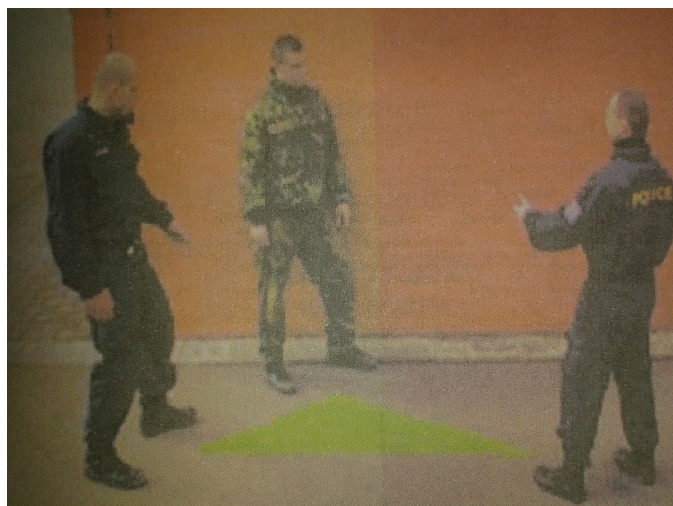
Obrázek 2. - Trojúhelníkové rozestavení hlídky
