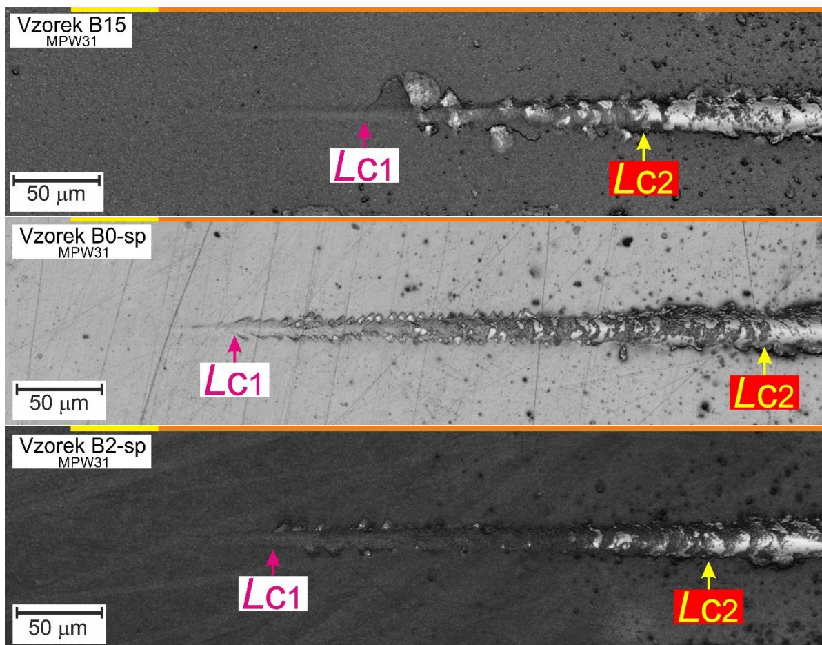
Obrázek 20: Grafické záznamy dílčích vrypů vzorků „B15“, „B0-sp“ a „B2-sp“
