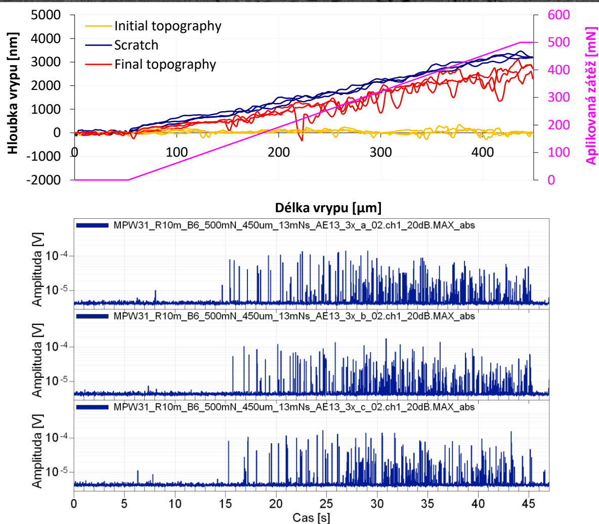
Obrázek 14: Grafické záznamy vrypů, záznam detekované hloubky a záznamy akustických emisí vzorku B6
