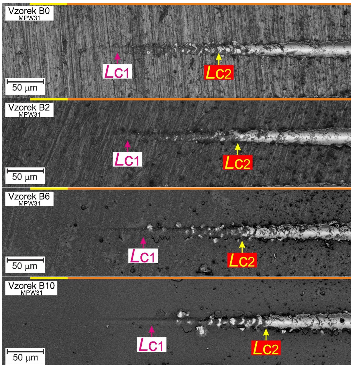
Obrázek 19: Grafické záznamy dílčích vrypů vzorků „B0“, „B2“, „B6“ a „B10“
