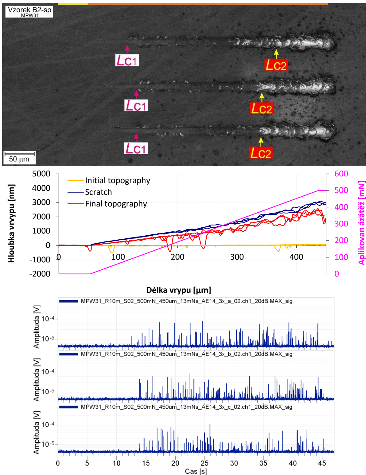
Obrázek 18: Grafické záznamy vrrpů, záznam detekované hloubky a záznamy akustických emisí vzorku B2-sp
