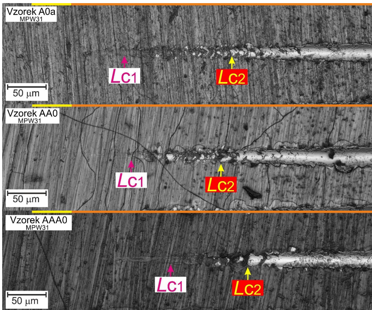
Obrázek 21: Grafické záznamy dílčích vrypů vzorků „A0a“, „AA0“ a „AAA0“
