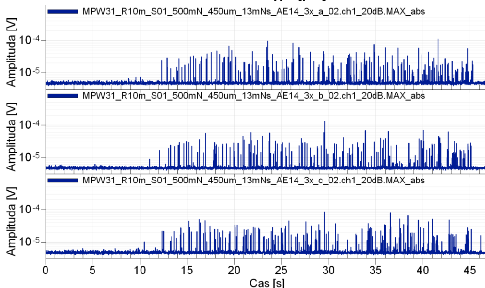
Obrázek 17: Grafické záznamy vrypů, záznam detekované hloubky a záznamy akustických emisí vzorku B0-sp
