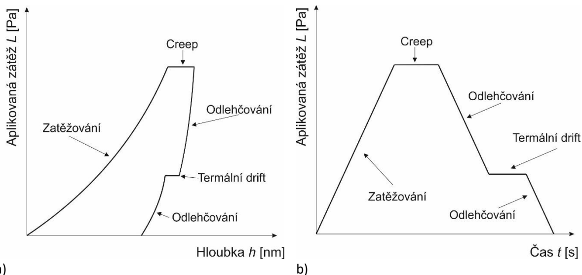
Obrázek 1: a) graf průběhu jednoho cyklu indentační zkoušky vzhledem k hloubce h ; b) vzhledem k času t
