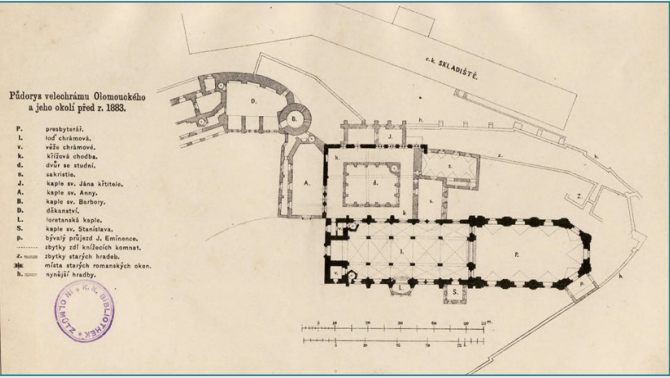
Půdorys velechrámu Olomouckého a jeho okolí před r. 1883 [OH8]
