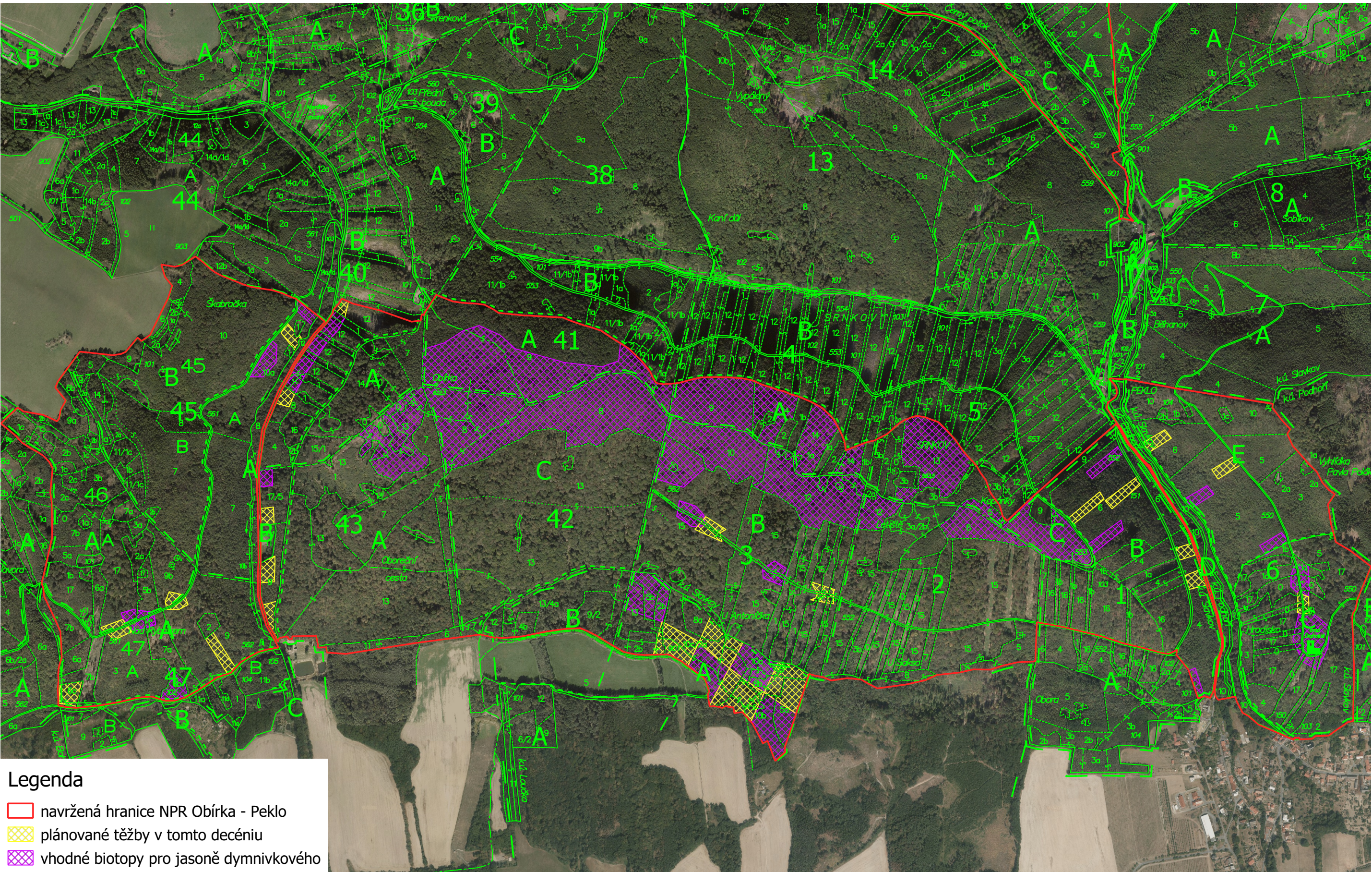
mapa č. 14: Mapa predikce výskytu vhodných biotopů pro jasoně dymnivkového ( Parnassius mnemosyne ) pro 5. decénium
