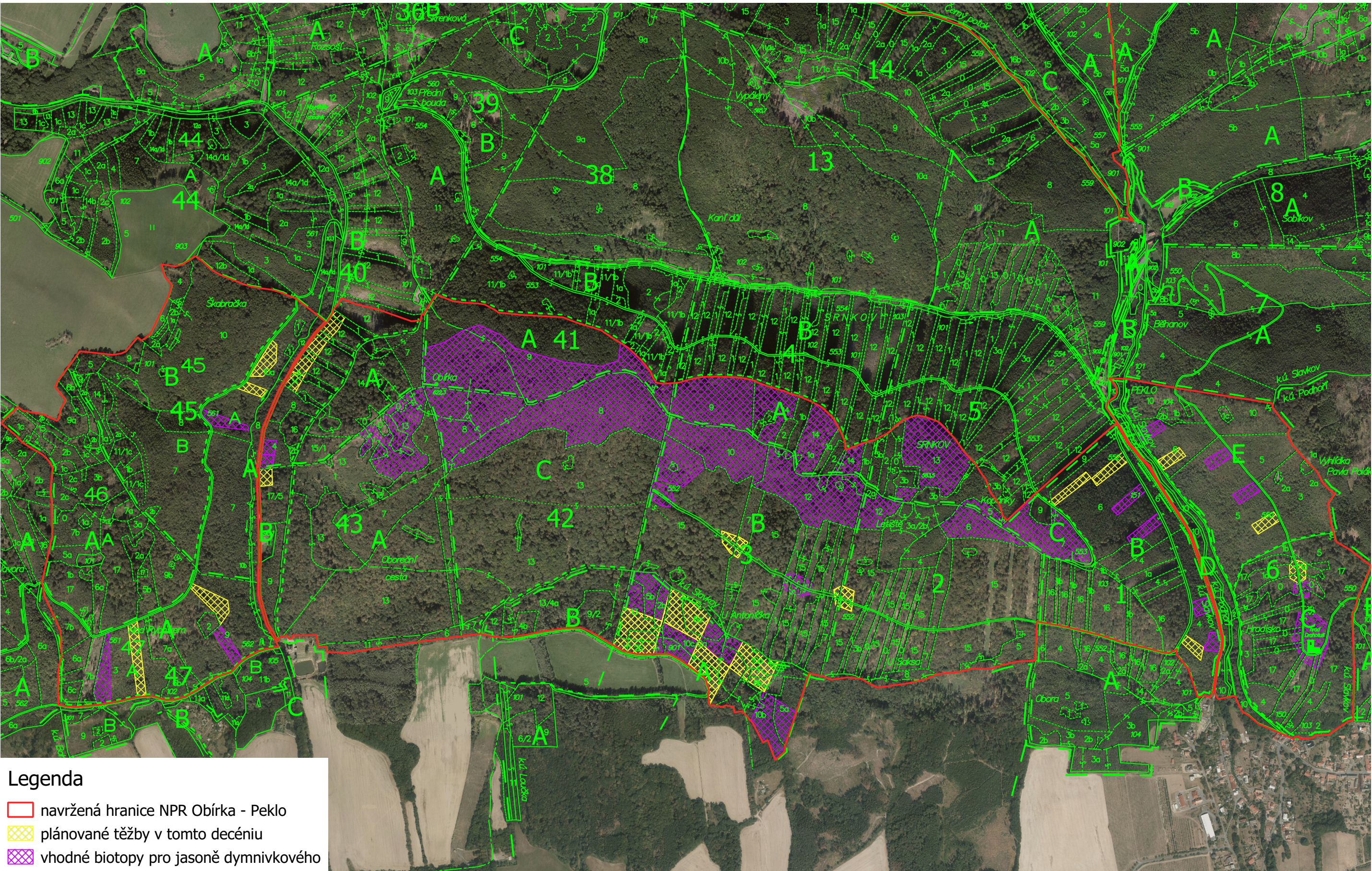
mapa č. 17: Mapa predikce výskytu vhodných biotopů pro jasoně dymnivkového ( Parnassius mnemosyne ) pro 8. decénium
