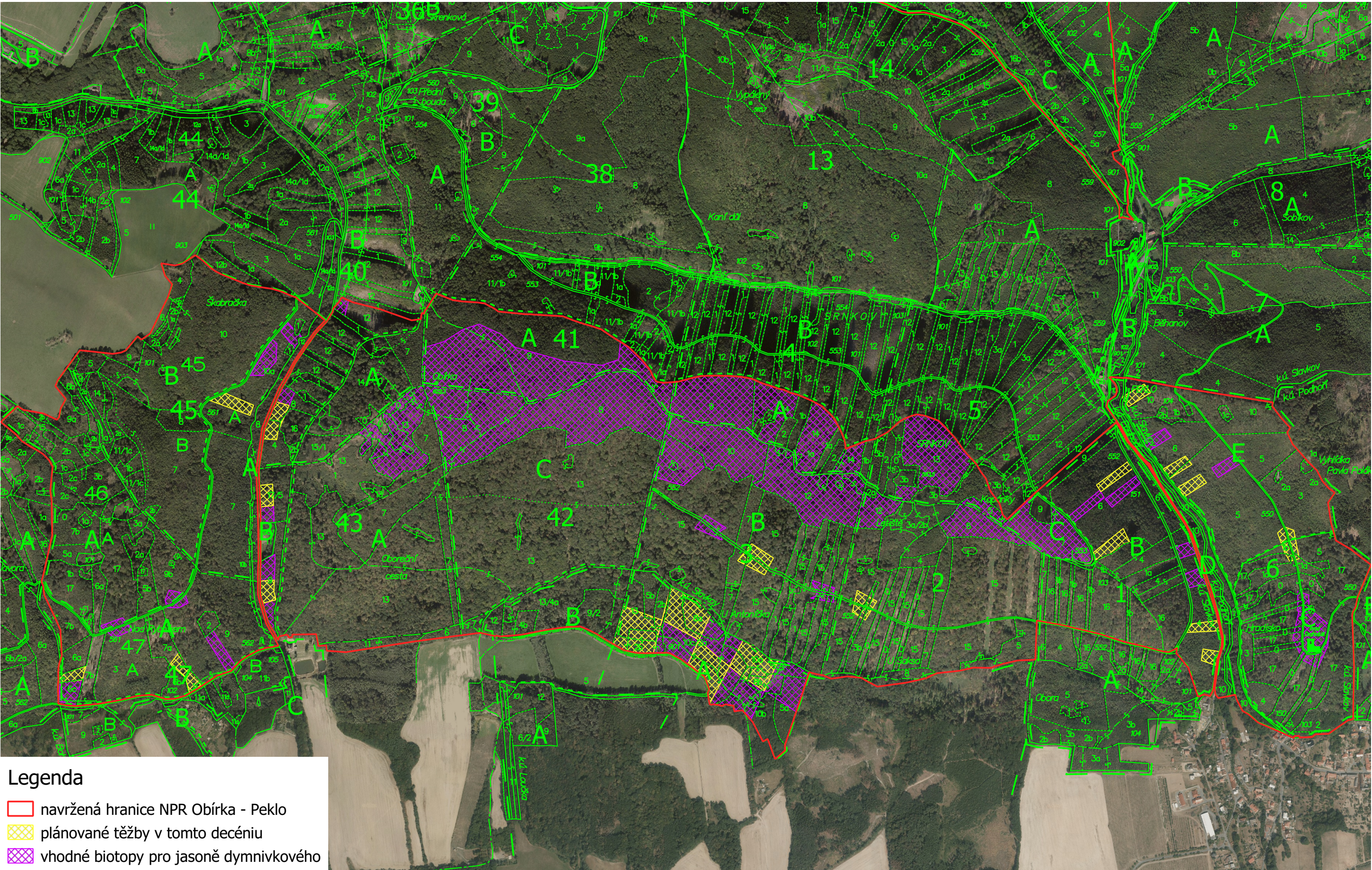
mapa č. 15: Mapa predikce výskytu vhodných biotopů pro jasoně dymnivkového ( Parnassius mnemosyne ) pro 6. decénium
