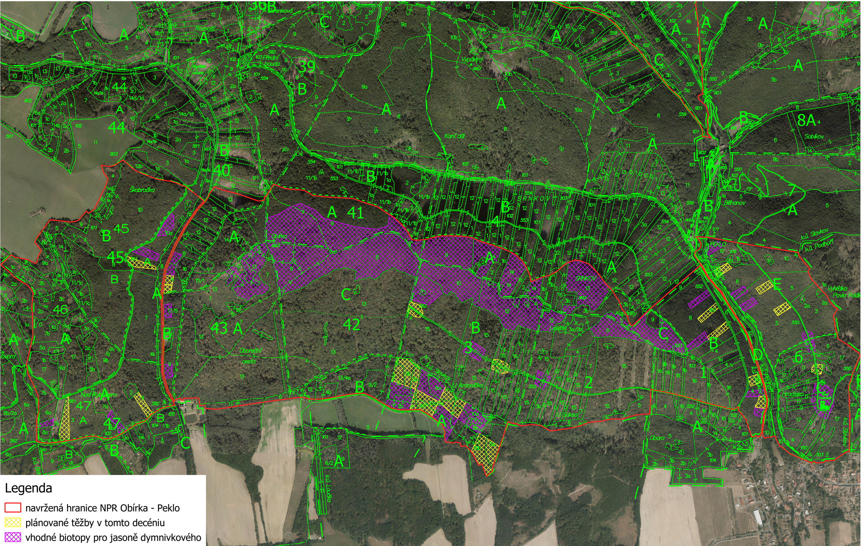
mapa č. 16: Mapa predikce výskytu vhodných biotopů pro jasoně dymnivkového ( Parnassius mnemosyne ) pro 7. decénium
