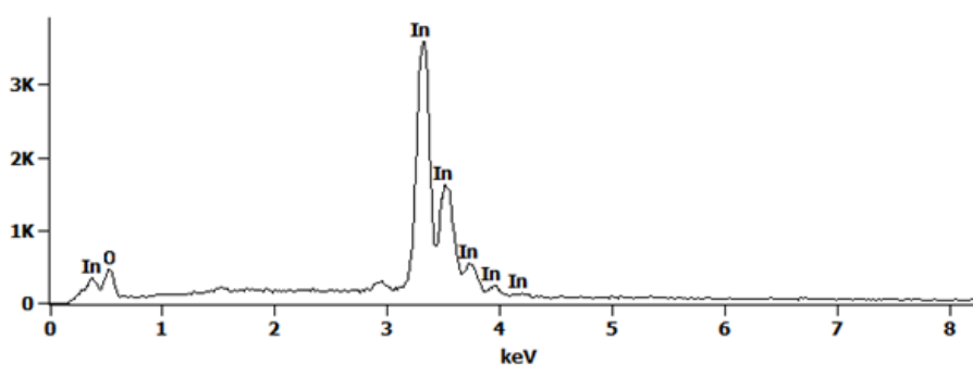
Obrázek 4: EDS spektrum \text{In}_2\text{O}_3 – 500
