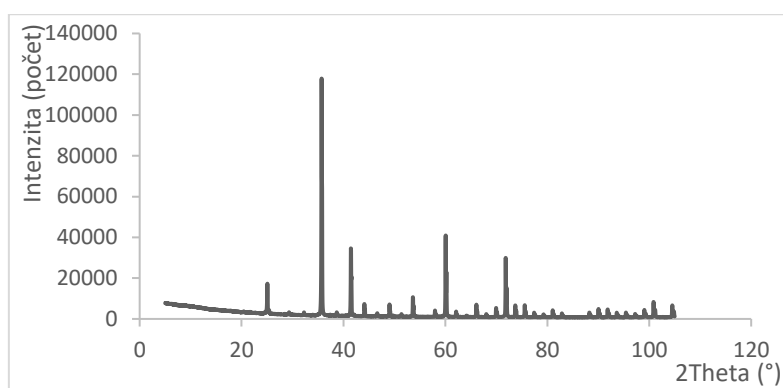
Obrázek 1: XRD spektrum referenčního \text{In}_2\text{O}_3
