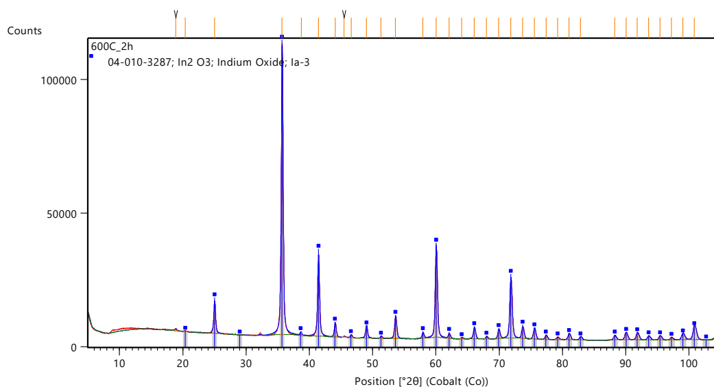
Obrázek 5: XRD spektrum \text{In}_2\text{O}_3 – 600
