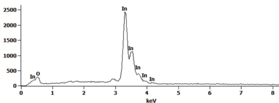
Obrázek 2: EDS spektrum \text{In}_2\text{O}_3 – 300
