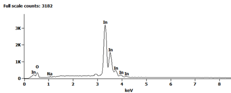
Obrázek 5: EDS spektrum In 2 O 3 – 600
