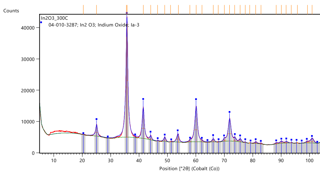
Obrázek 2: XRD spektrum \text{In}_2\text{O}_3 – 300
