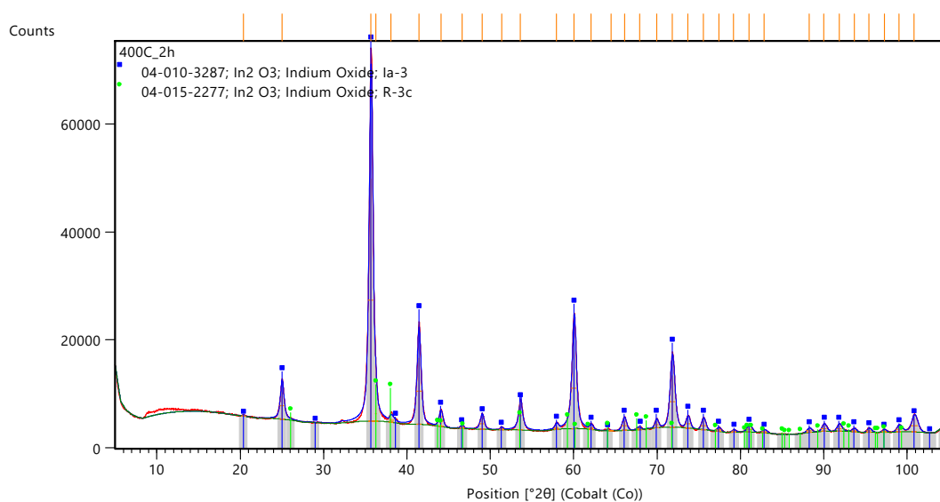
Obrázek 3: XRD spektrum \text{In}_2\text{O}_3 – 400
