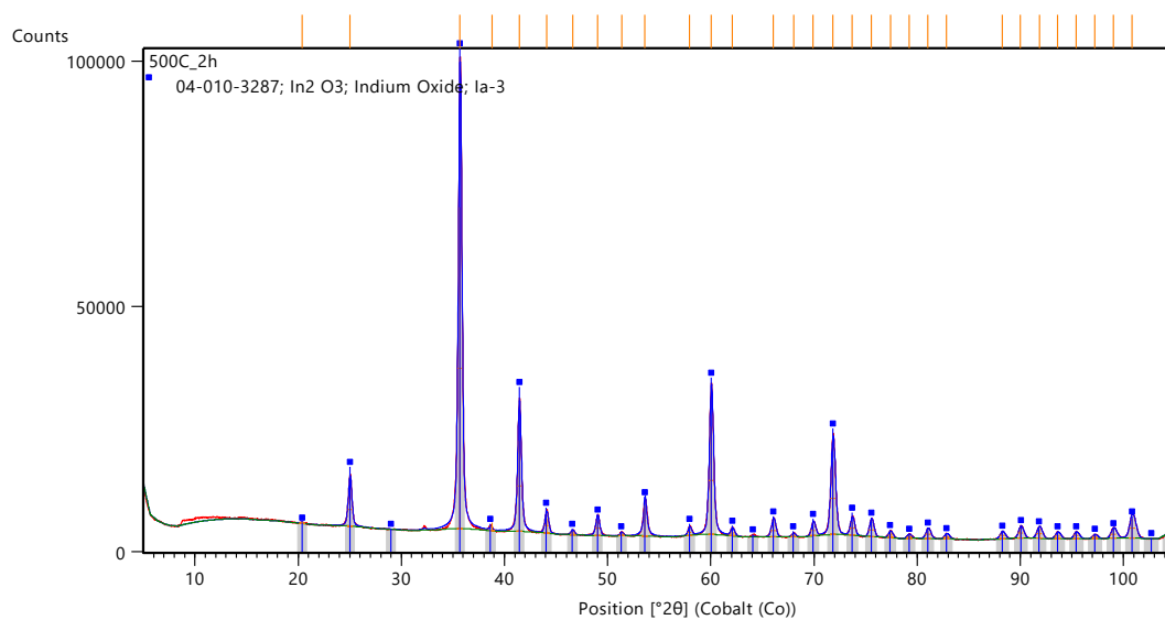
Obrázek 4: XRD spektrum \text{In}_2\text{O}_3 – 500
