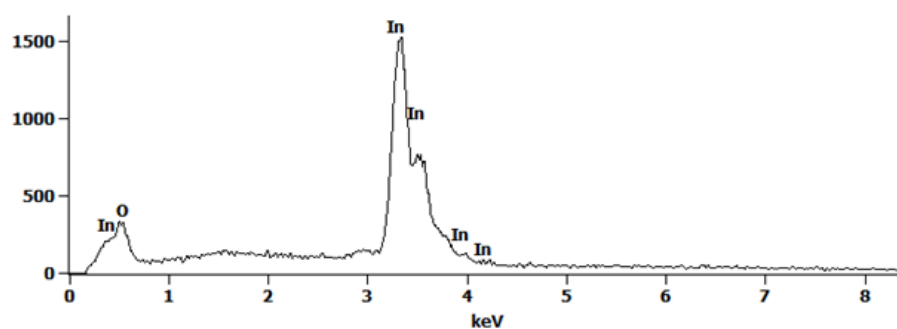
Obrázek 1: EDS spektrum referenčního \text{In}_2\text{O}_3
