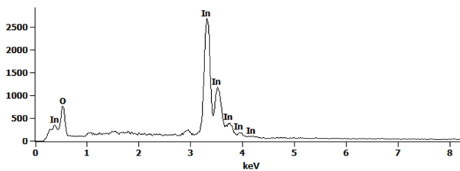
Obrázek 3: EDS spektrum \text{In}_2\text{O}_3 – 400
