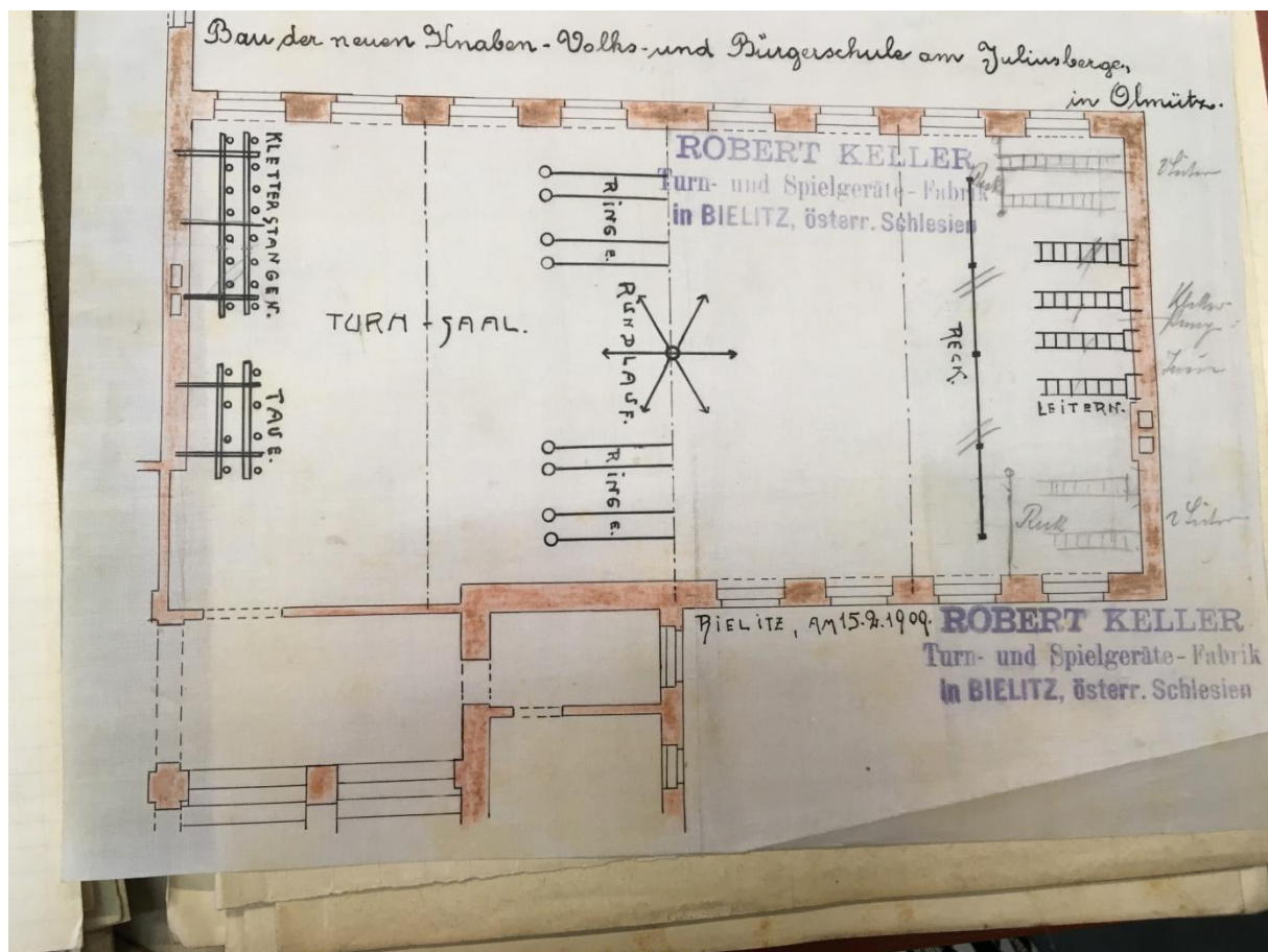
Obr. 3: Plán rozmístění cvičebního nářadí v tělocvičně
