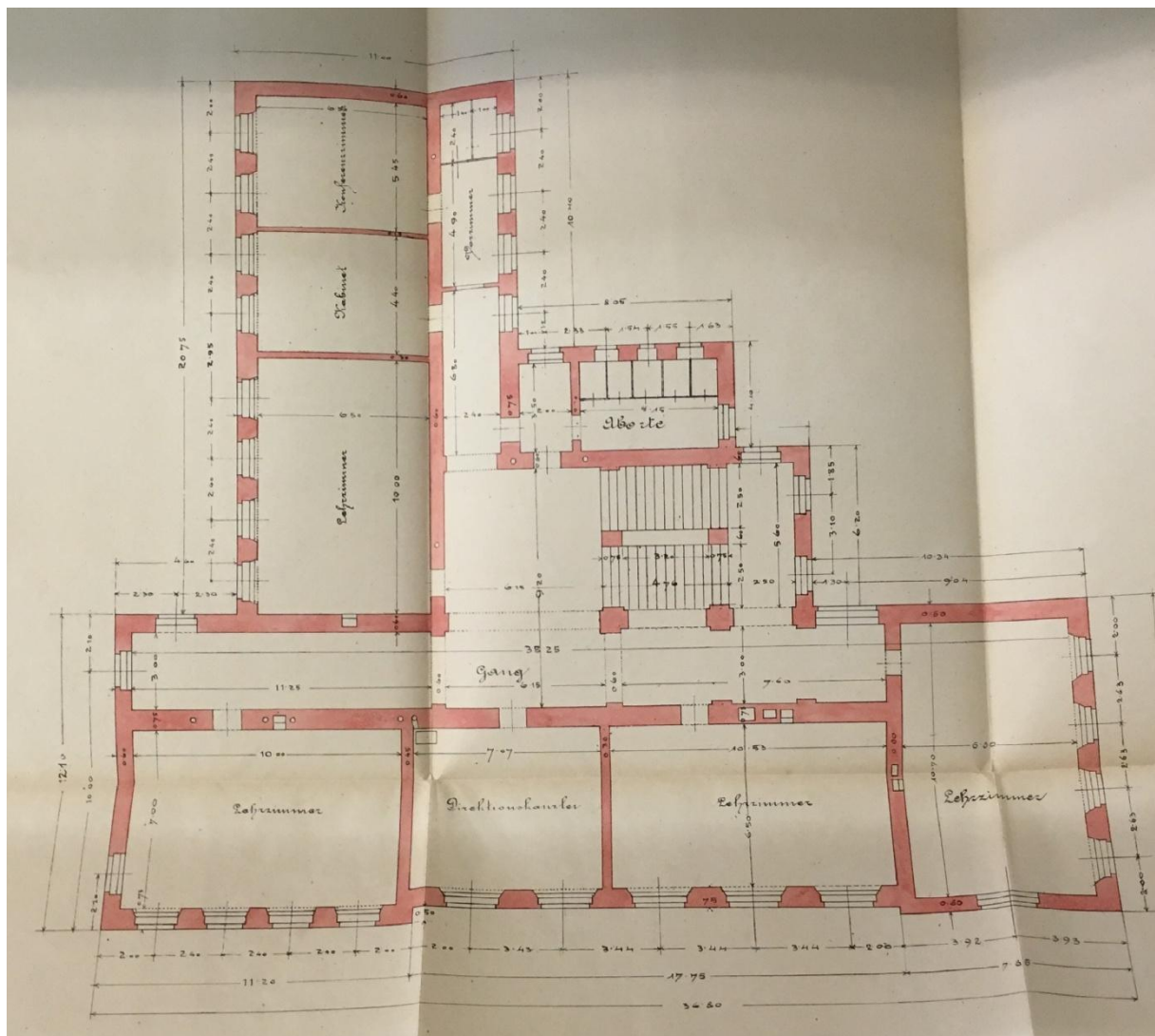
Obr. 1: Rozložení místností v 1. patře budovy
