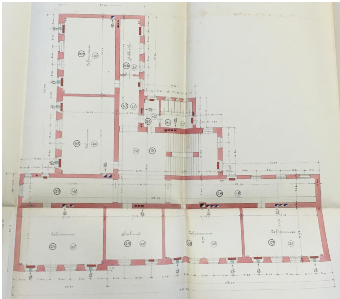
Obr. 2: Umístění topení ve 2. patře
