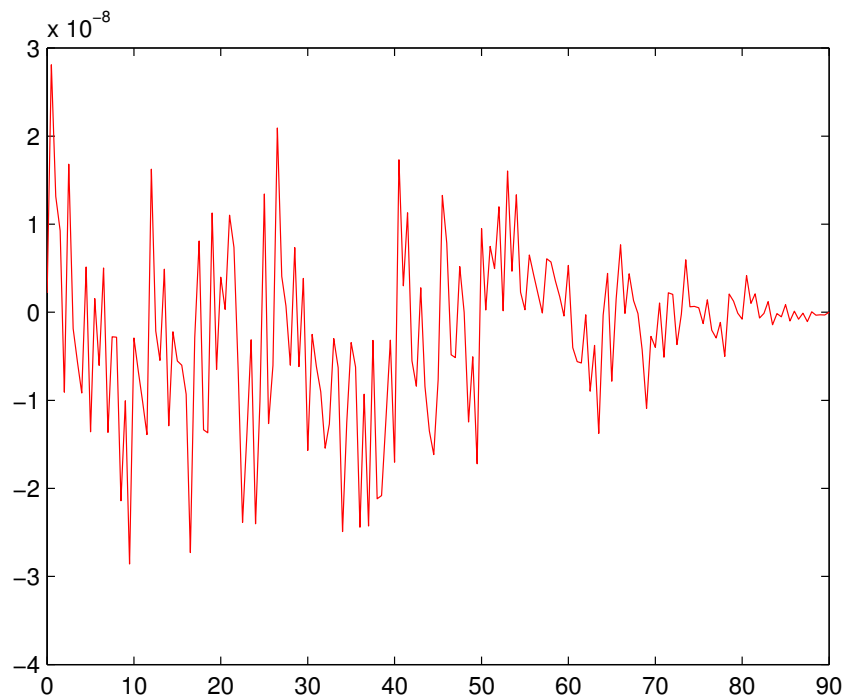
Obrázek 4: absolutní chyba
