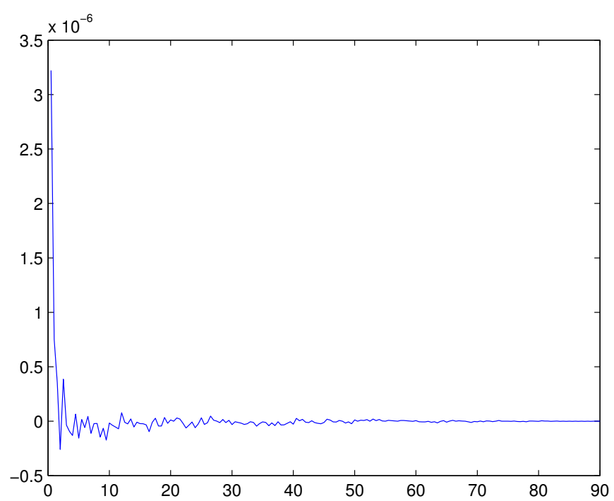
Obrázek 5: relativní chyba
