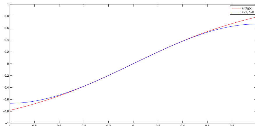
Obrázek 1: Arkustangens Taylorova polynomu řádu 3
