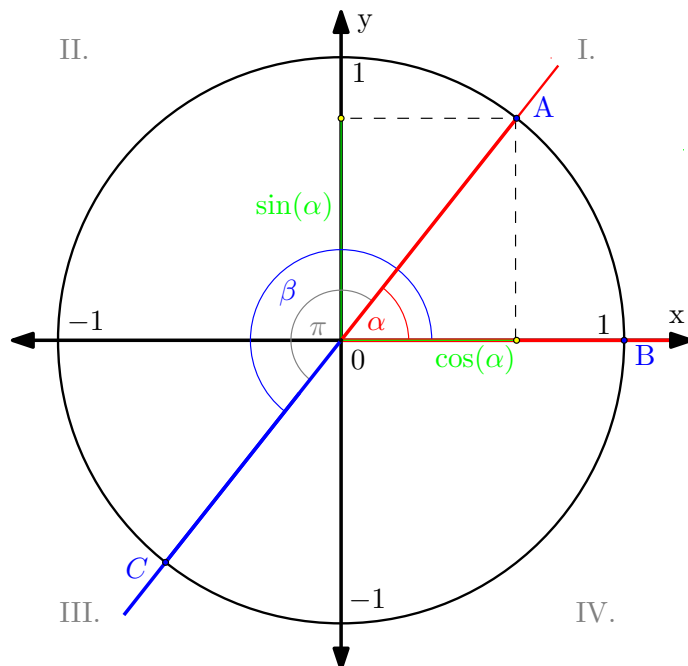
Obrázek 3: Jednotková kružnice
